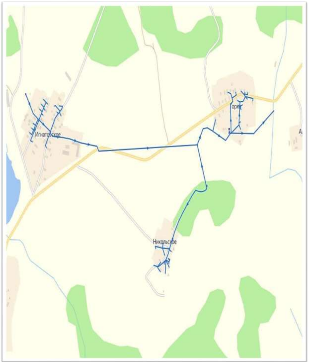
Рис.2. Схема водоснабжения д. Горка- д. Игнатовское.
