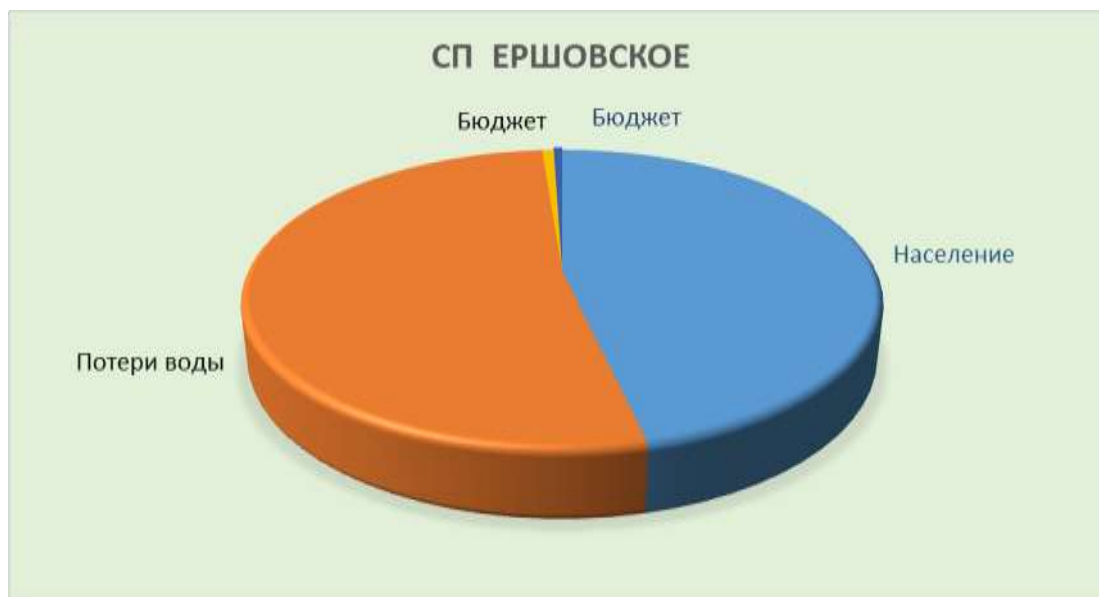
Рис.5. Баланс подачи и реализации воды в системе водоснабжения в Ершовском сельском поселении .
