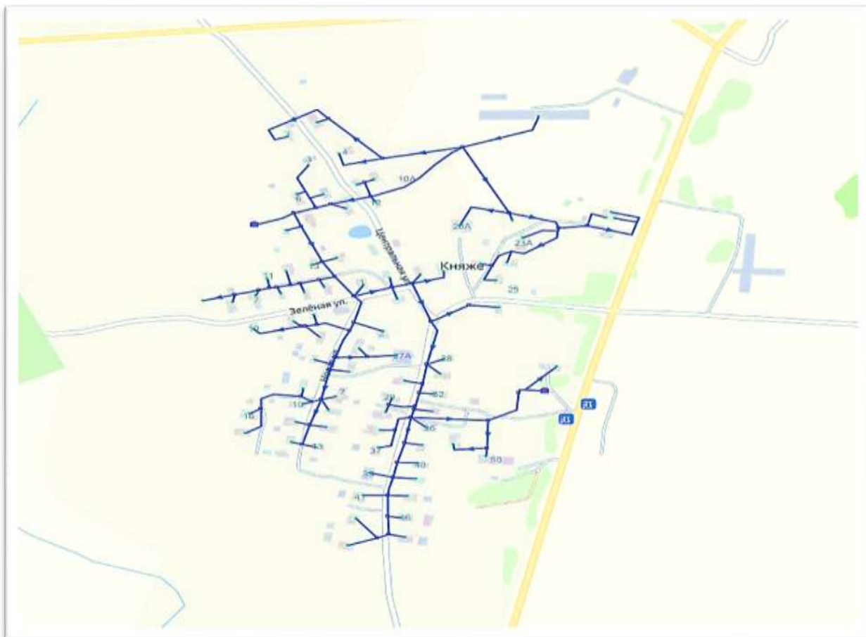
Рис.3. Схема водоснабжения Княже.
